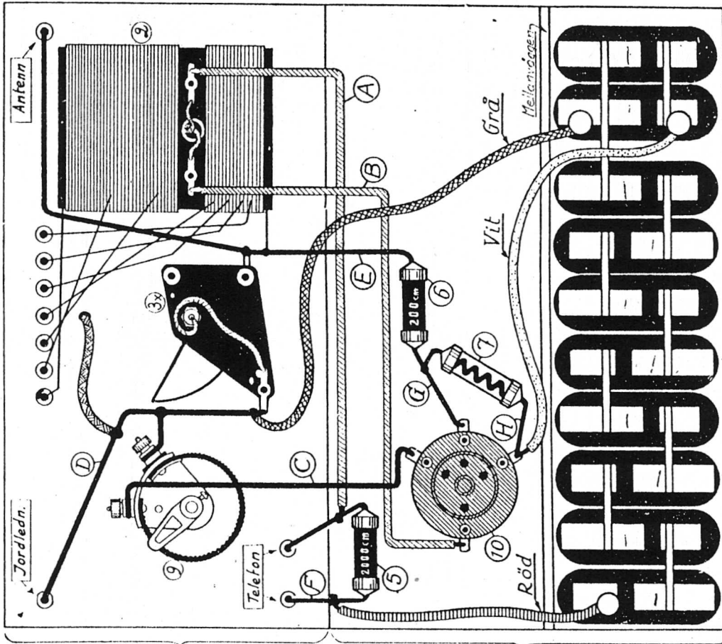
Kopplingsplan.
